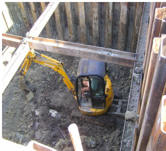
Hloubení štěrbinové nádrže
